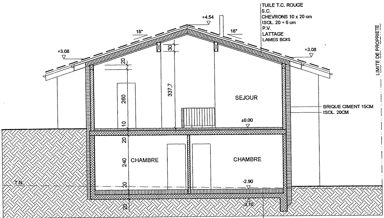
COUPE A-A
