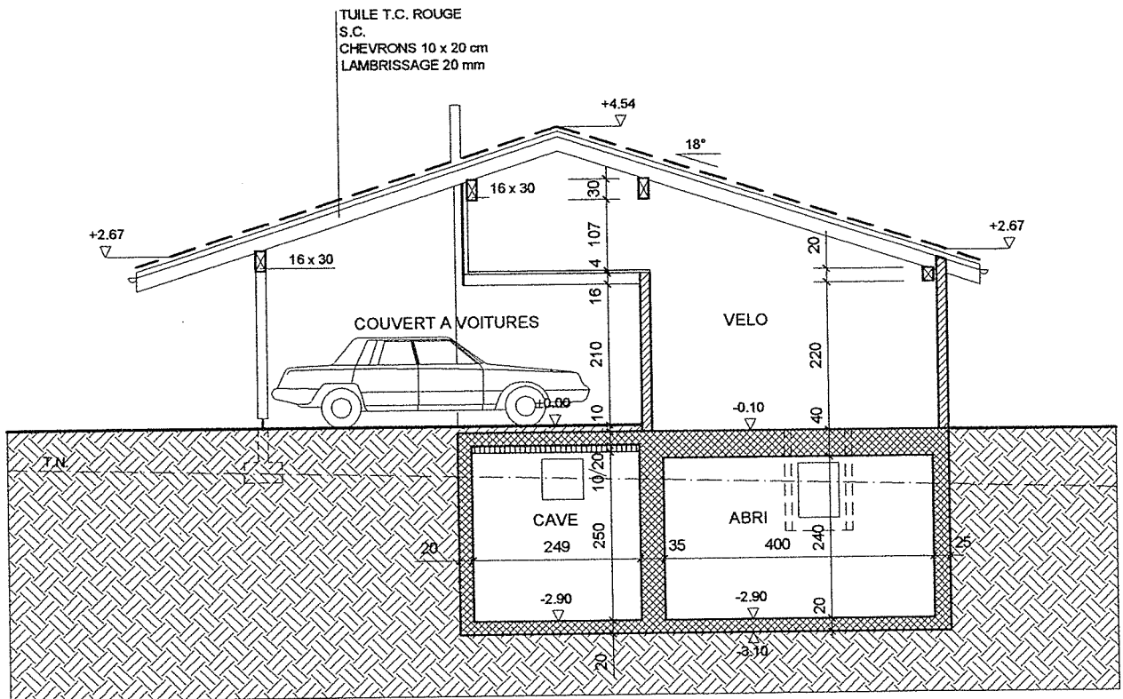
COUPE B-B
