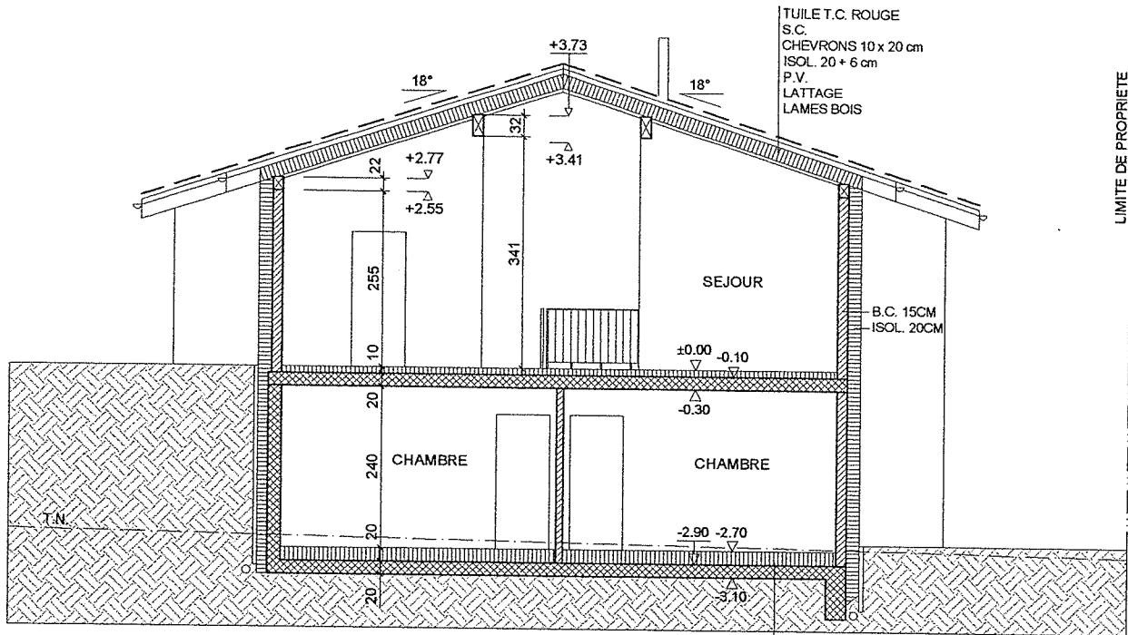
COUPE A-A
