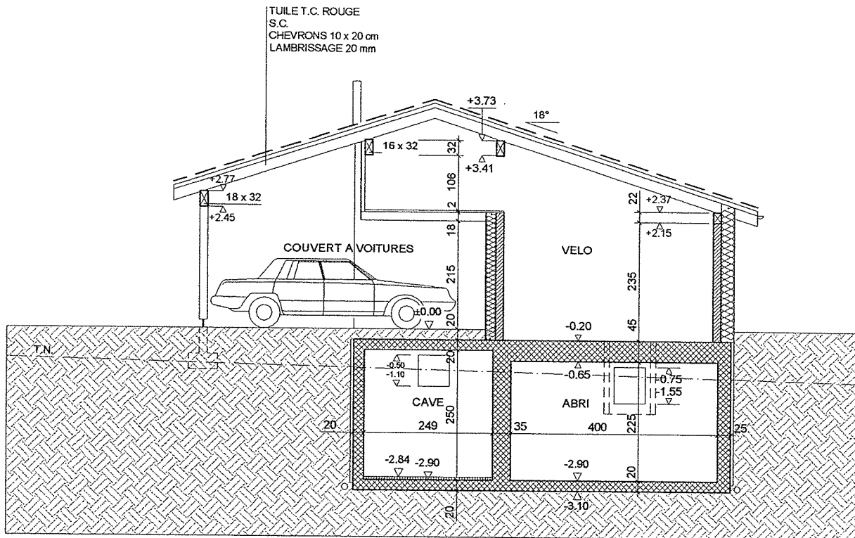
COUPE B-B
